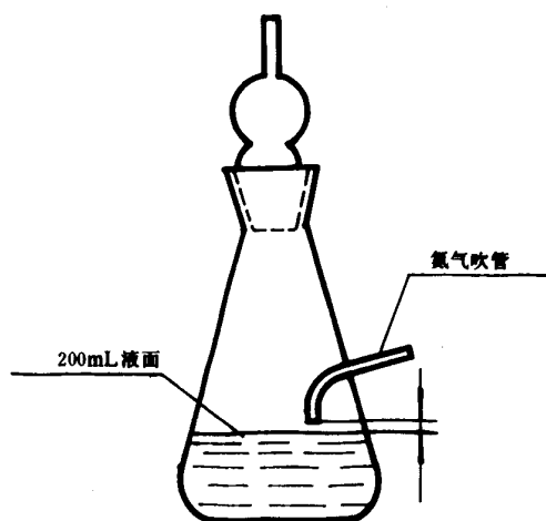
锥形瓶图
